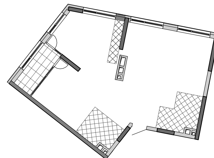
План квартири без перегородок
