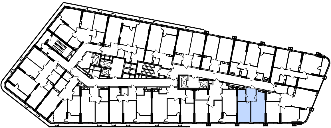
План поверху
